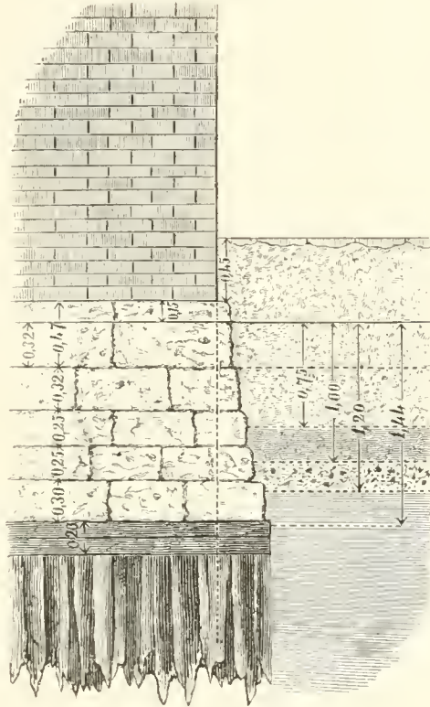
Unterbau des Markusdoms.
